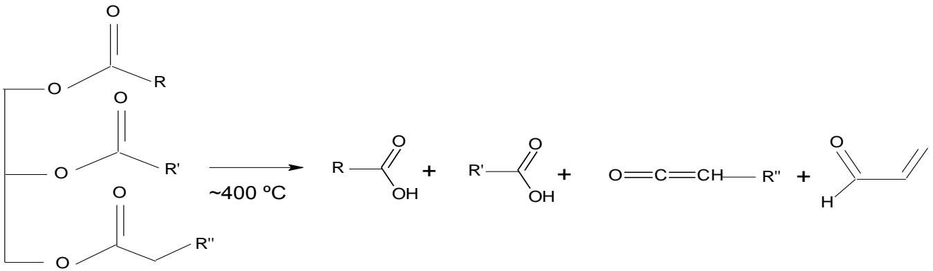
Figura 3.3 -Reação Global do Craqueamento Primário.
