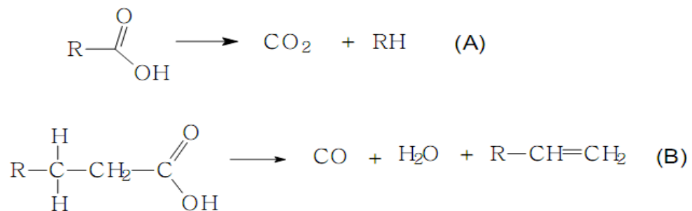
Figura 3.4 - Mecanismos da desoxigenação dos ácidos carboxílicos: (A) descarboxilação e (B) descarbonilação.
