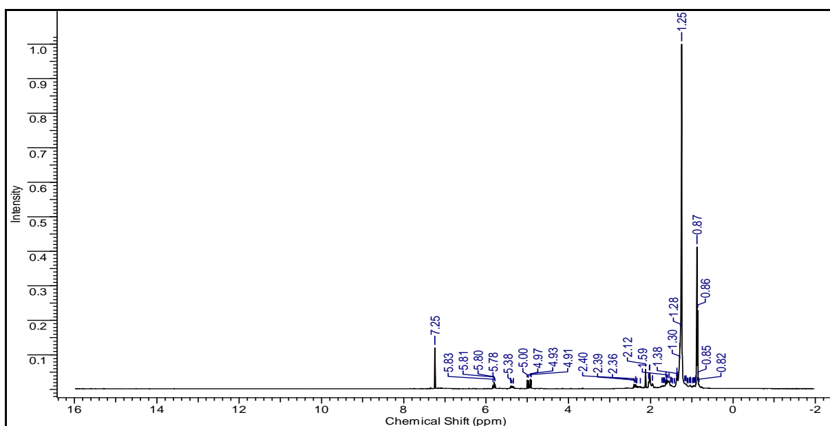
Figura 5.7- Espectro de RMN ^1\text{H} do PLO produzido na Unidade Piloto de Craqueamento utilizando o teor de 10% de \text{Na}_2\text{CO}_3 .
