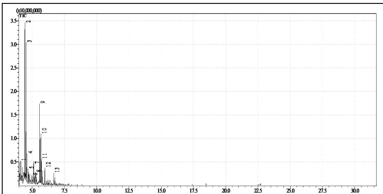
Figura 5.13- Cromatograma do querosene verde obtido na unidade de destilação em escala de bancada.
