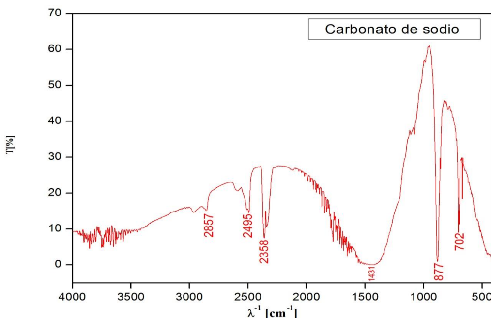
Figura 5.3- Espectro de infravermelho do carbonato de sódio.
