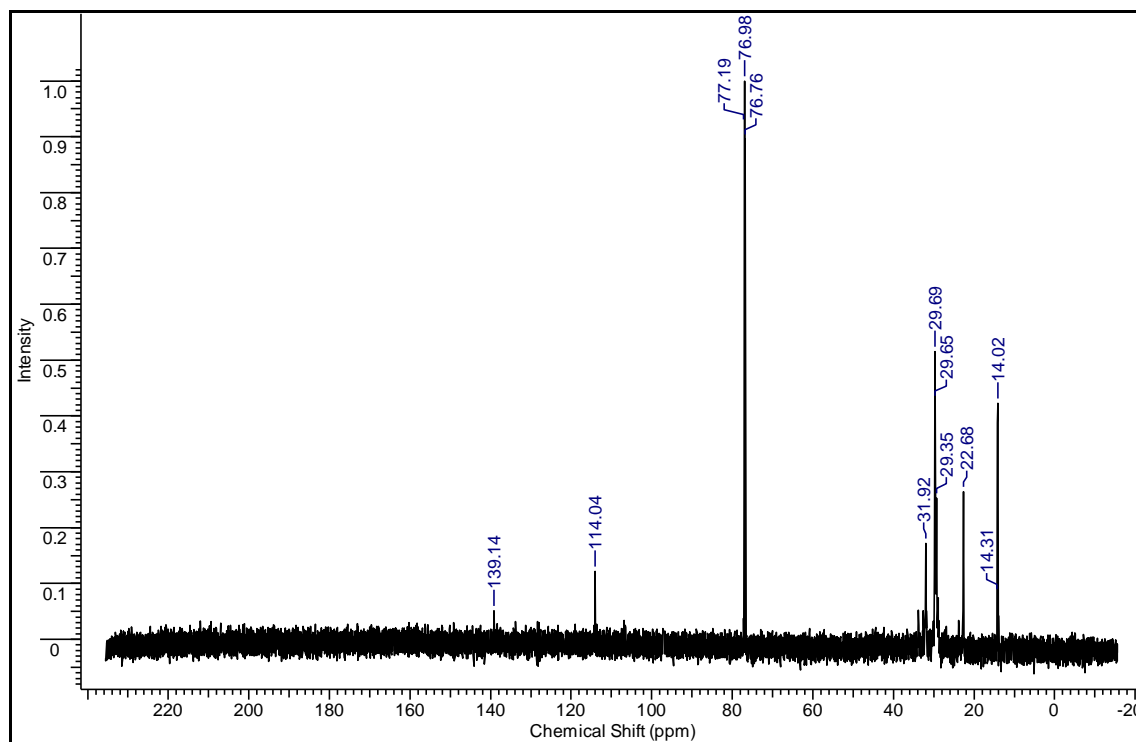
Figura 5.17- Espectro de RMN ^{13}\text{C} do Diesel Verde Pesado produzido na Unidade de Destilação em Escala de Bancada.
