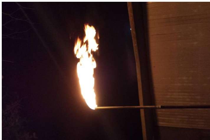
Figura 4.35- Queima dos Gases Não Condensáveis.
