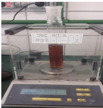
Figura 4.16- Gordura e Catalisador sendo pesados e colocados no Reator. Fonte: O autor.
