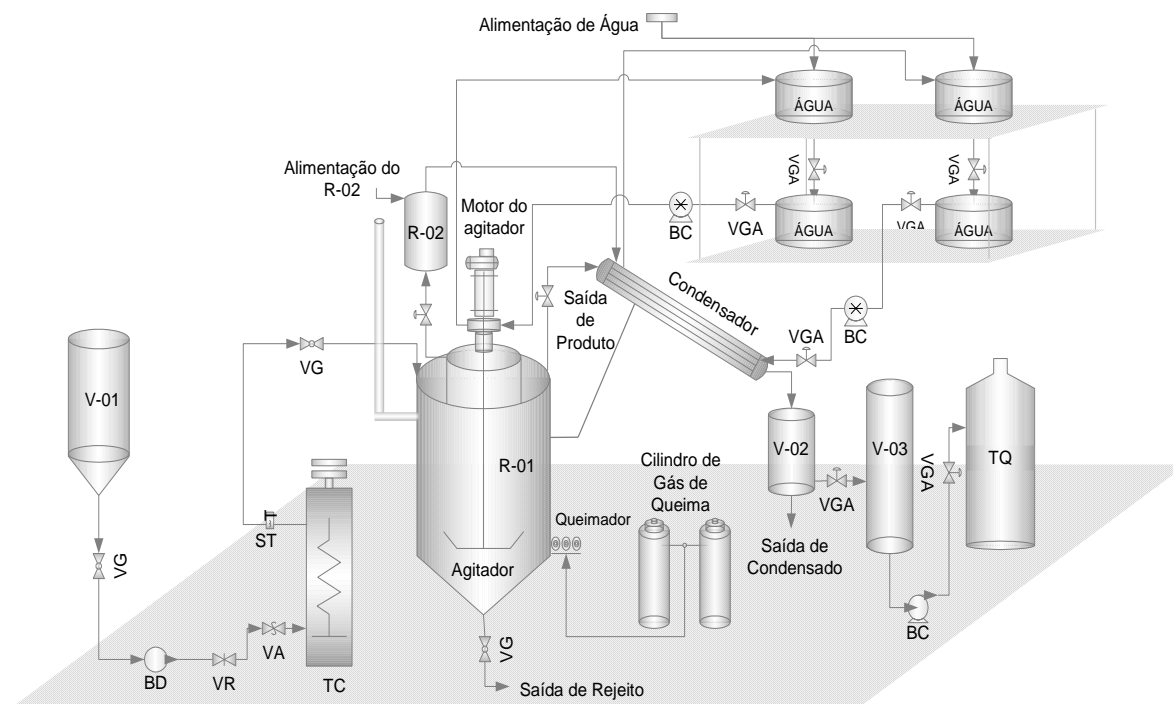
Figura 4.37- Fluxograma da Unidade Piloto de Craqueamento. Fonte: MOTA, 2013.
