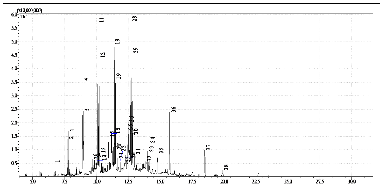
Figura 5.19- Cromatograma do diesel verde pesado obtido na unidade de destilação em escala de bancada.
