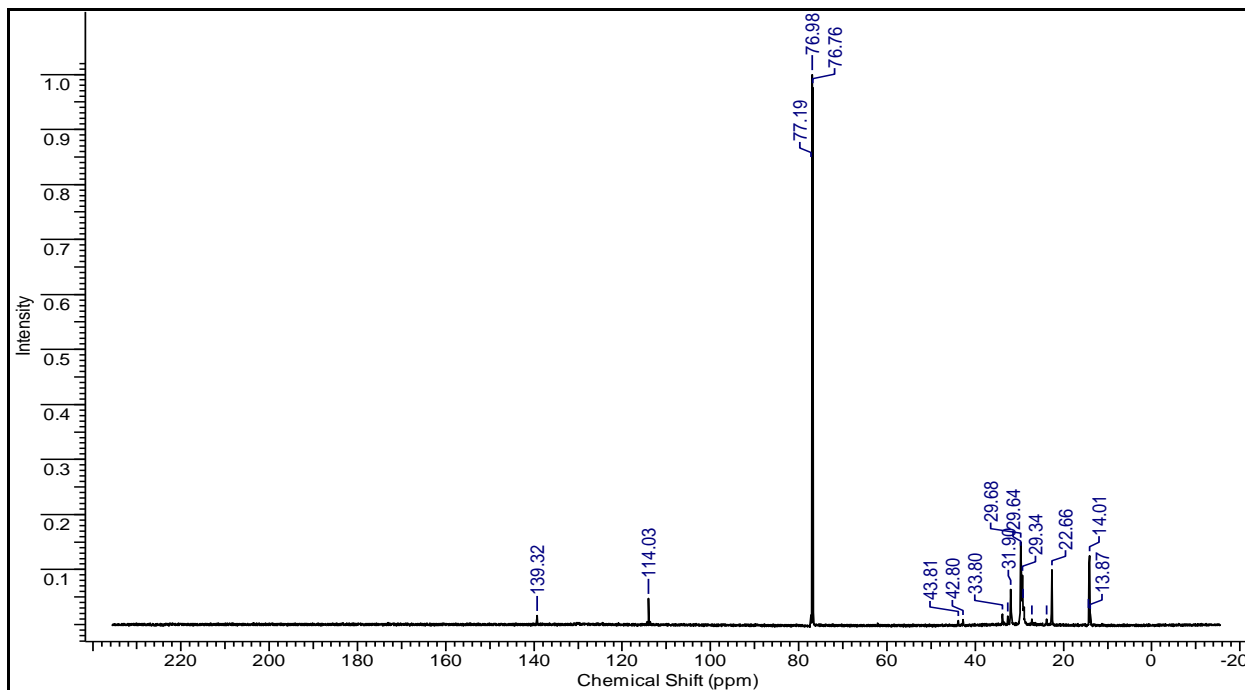
Figura 5.6- Espectro de RMN ^{13}\text{C} do PLO produzido na Unidade Piloto de Craqueamento utilizando o teor de 10% de \text{Na}_2\text{CO}_3 .
