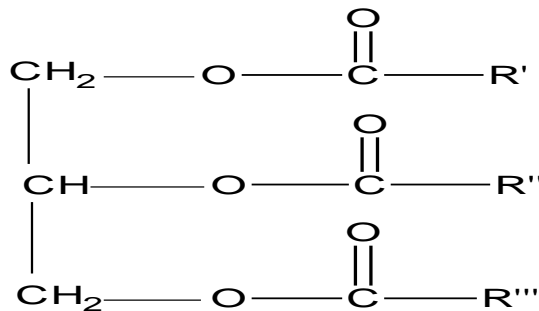
Figura 3.2- Representação de uma Molécula de Triglicerídeo.
